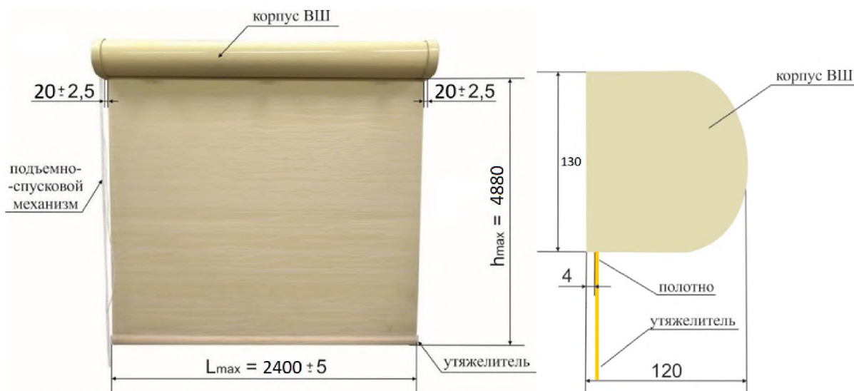
Рисунок 2 – Внешний вид ВШ-5 (размеры указаны в мм)
