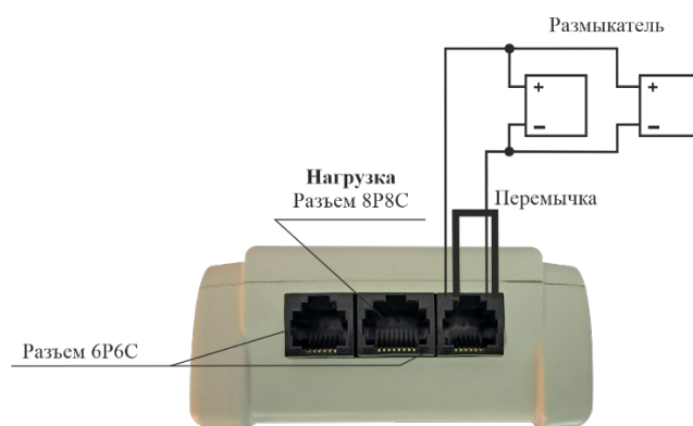
Рисунок 7 – Схема подключения размыкателей
