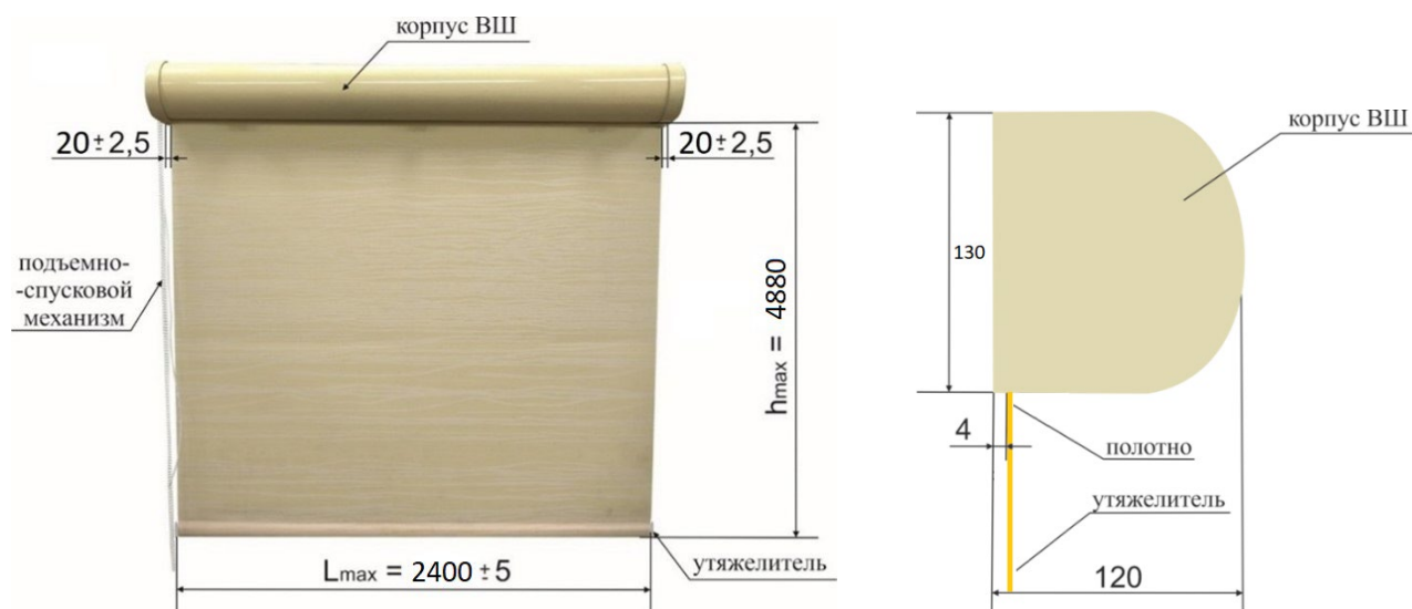
Рисунок 2 – Внешний вид ВШ-5 (размеры указаны в мм)
