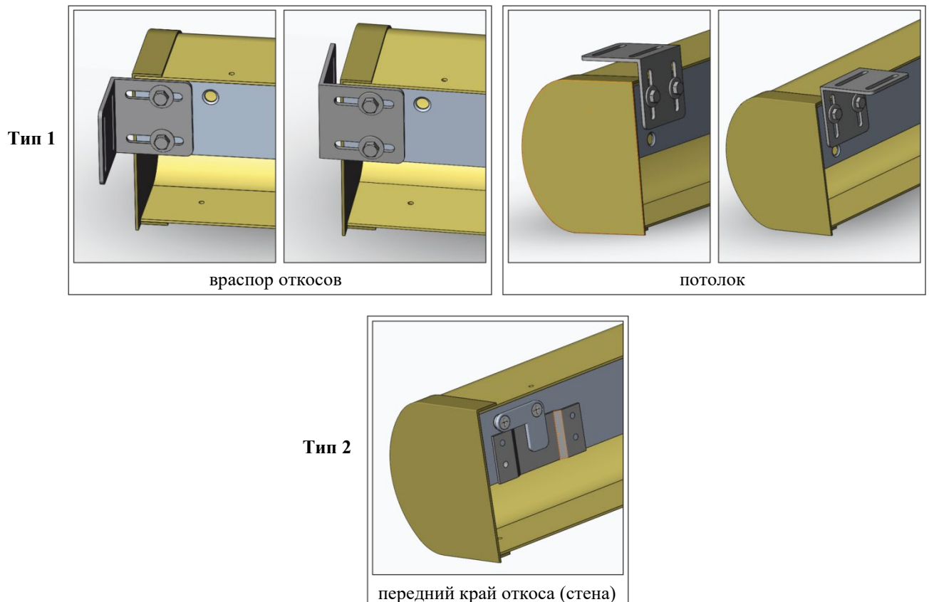
Рисунок 3 – Типы крепления ВШ
