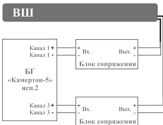
Рисунок 6 – Схема подключения ВШ-1/ВШ-2/ВШ-2и
