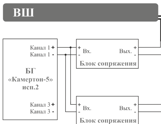
Рисунок 6 – Схема подключения ВШ-1/ВШ-2/ВШ-2и
